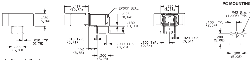
Actuator Shown In Pos. 1
